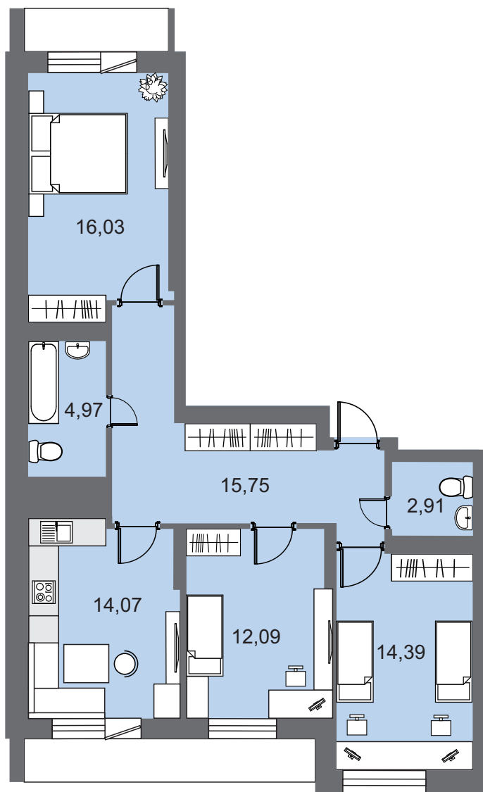
Типовая планировка с мебелью
